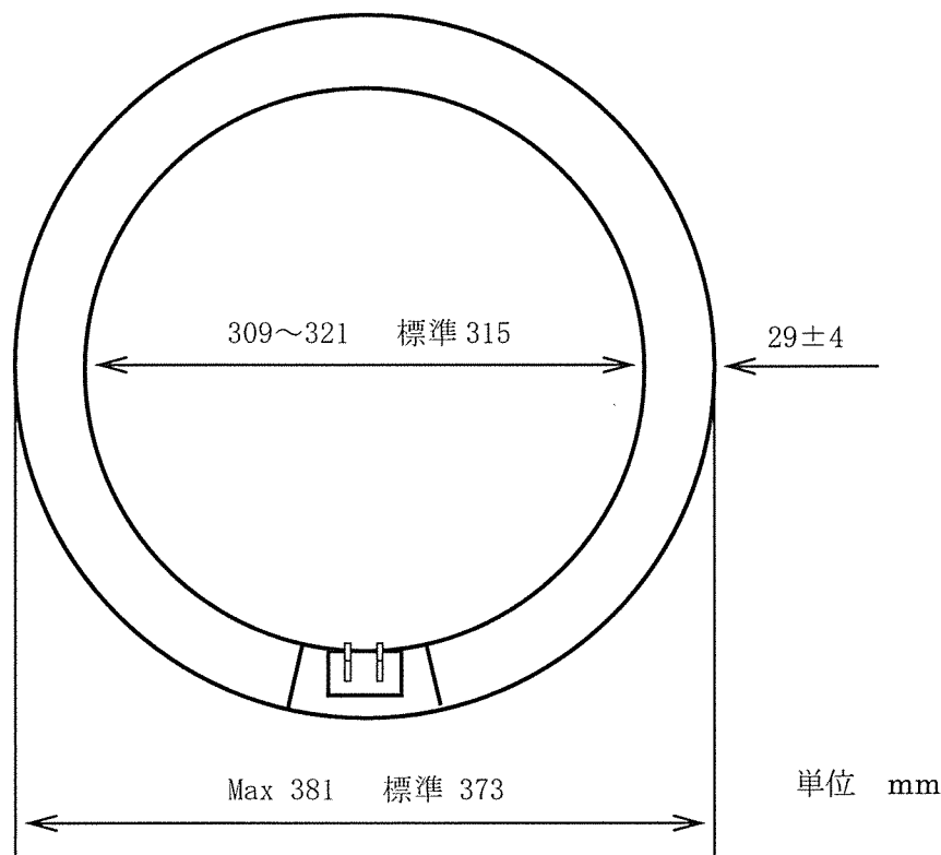
白色蛍光ランプ（環形）〈リングライト〉
